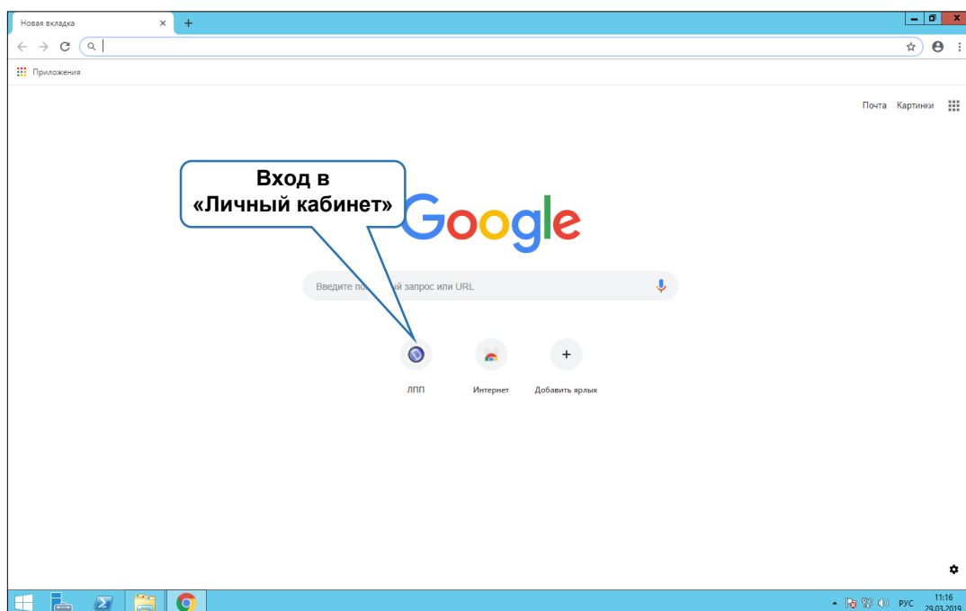
Рисунок 1 – Окно браузера
